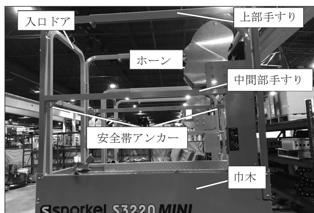
図8.14 - 作業床
