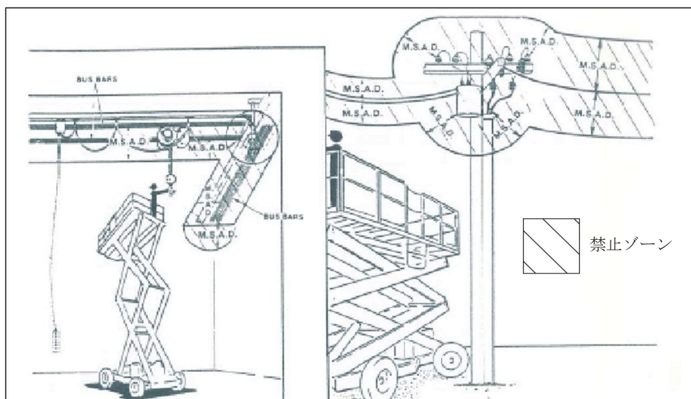
図3.1 - 最小離隔距離
