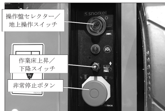
図8.8 - 下部操作盤
