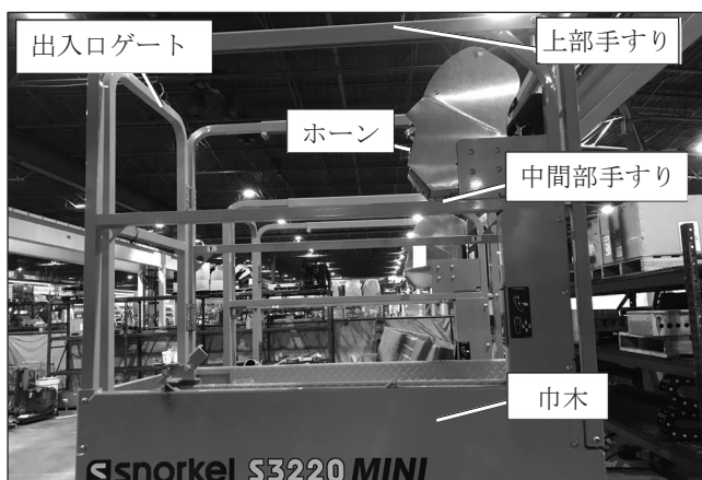
図4.7 - 作業床
