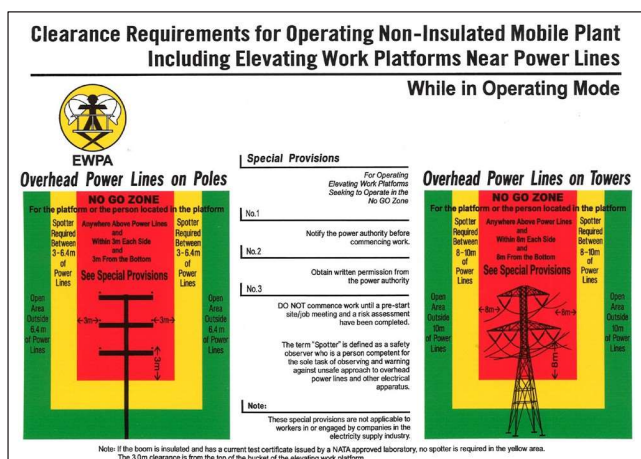
図3.2 - 最小離隔距離
