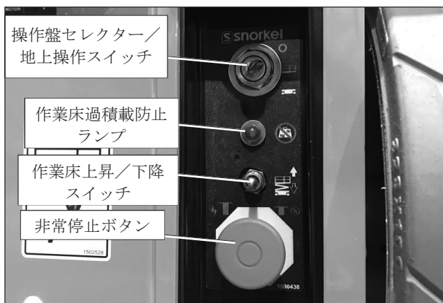
図4.1 - 下部操作盤
