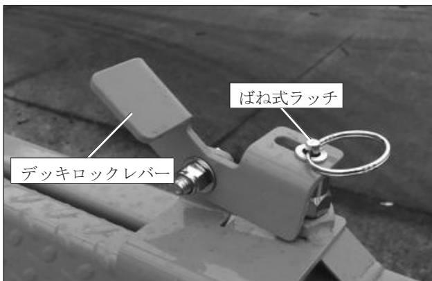
図9.4 - 作業床延長デッキロック
