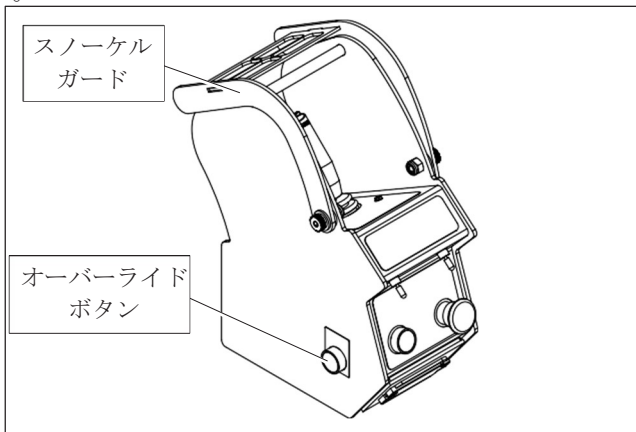
図7.5 - 上部操作盤
