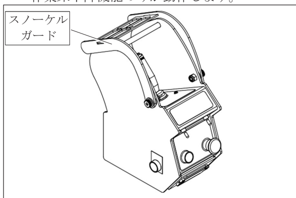
図4.9 - 上部操作盤
