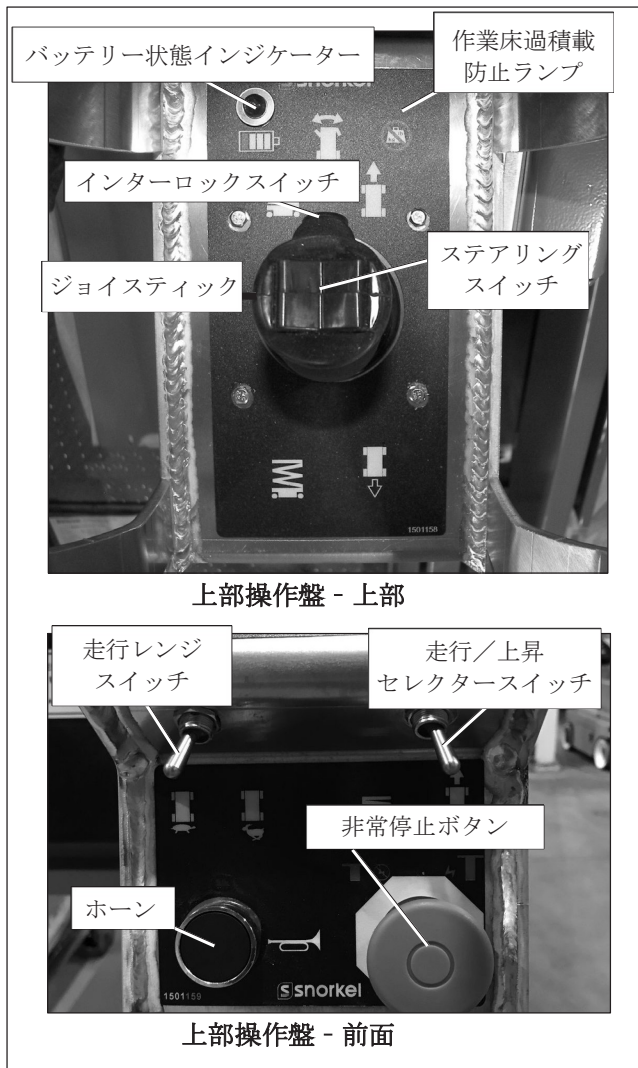
図7.3 - 上部操作盤
